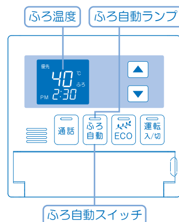
ふろリモコン表示部
