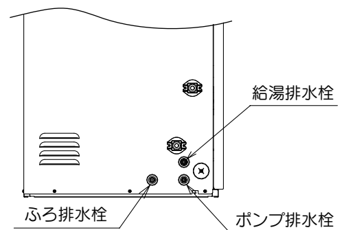
排水栓位置図
