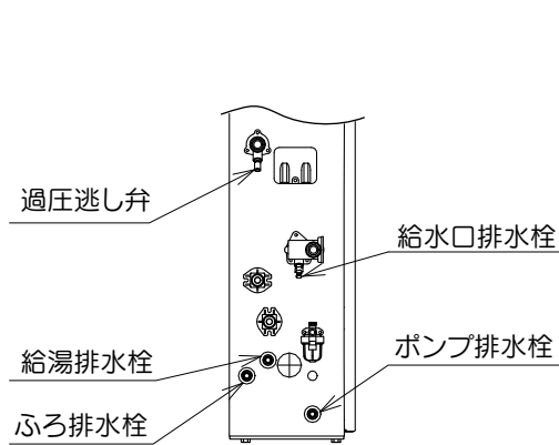
排水栓位置図
