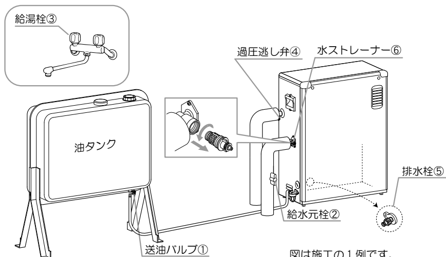
図は施工の1例です。 配管の形状などは実際と異なります。
